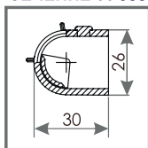
СЕЧЕНИЕ OZ 200
