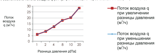
График. Зависимость потока воздуха q (м 3 /ч), протекающего через клапан VT 600, от разницы давления p(Па)
