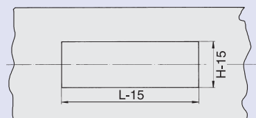
Сечение воздуховода
