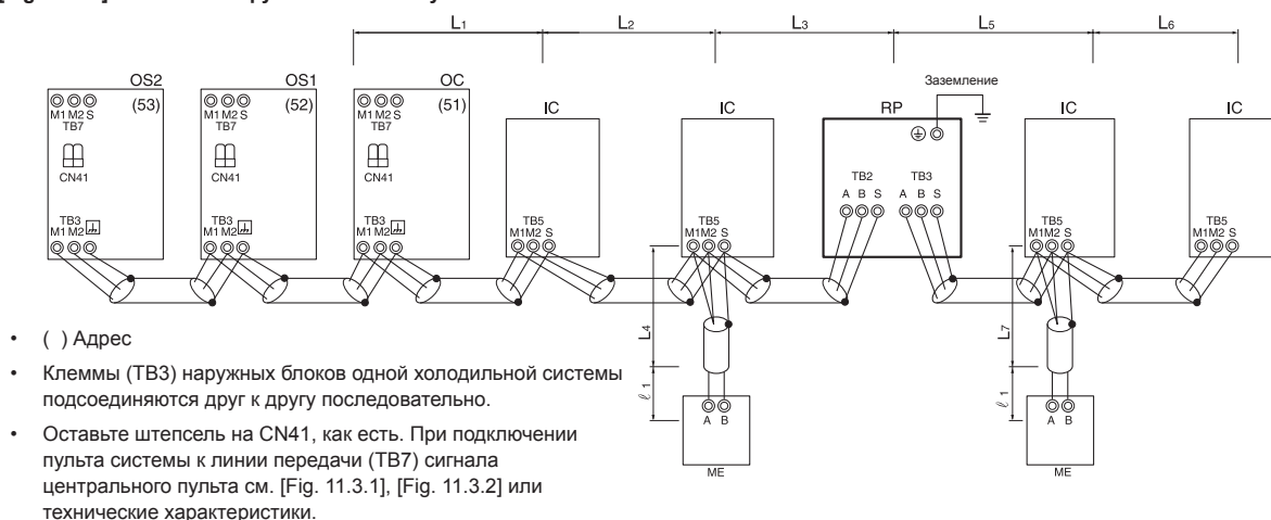
[Fig. 11.3.3] Сочетание наружных блоков и усилителя сигнала
