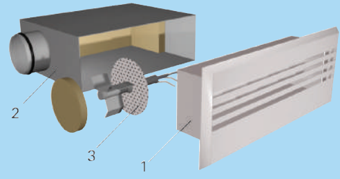
TLB/A (façade) + TLB/E (plénum Ø latéral)
