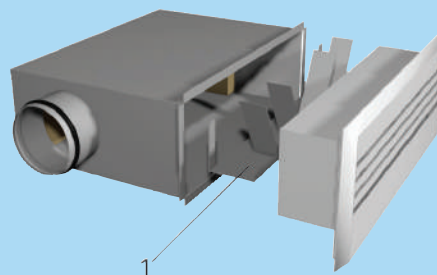
TLB/A (façade) + TLB/E (plénum Ø latéral)
