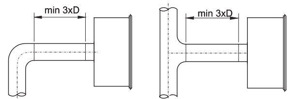
TLB/A (façade) + TLB/E (plénum Ø latéral)
