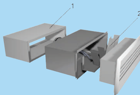
TLB/A (façade) + TLB/B (plénum Ø arrière)
