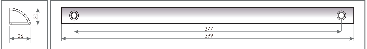
СЕЧЕНИЕ OZ 100
