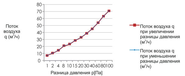
График 7. Зависимость потока воздуха q ( \text{м}^3/\text{ч} ), протекающего через клапан VT 701, от разницы давления p (Па)
