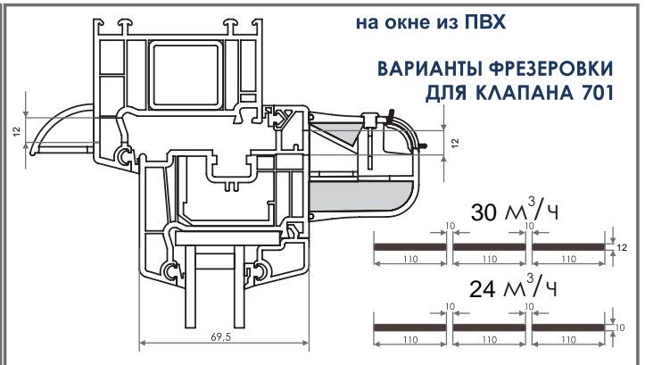
ВАРИАНТЫ ФРЕЗЕРОВКИ ДЛЯ КЛАПАНА 701
