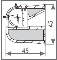
СЕЧЕНИЕ VT 300
