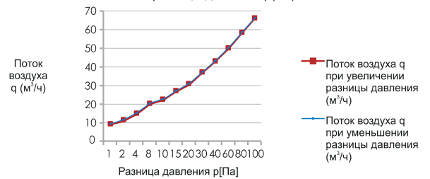
График 5. Зависимость потока воздуха q ( \text{м}^3/\text{ч} ), протекающего через клапан VT 301, от разницы давления p (Па)
