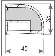
СЕЧЕНИЕ OZ 400
