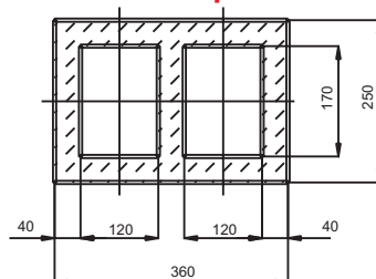
Bryza-120/170 на пустотелый вентиляционный блок типа "Schiedel" вертикальный
