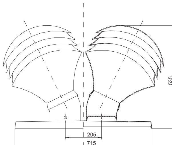
Дефлектор BRYZA-150/W2 в многосегментной системе
