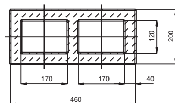
Bryza-120/170 на пустотелый вентиляционный блок типа "Schiedel" горизонтальный
