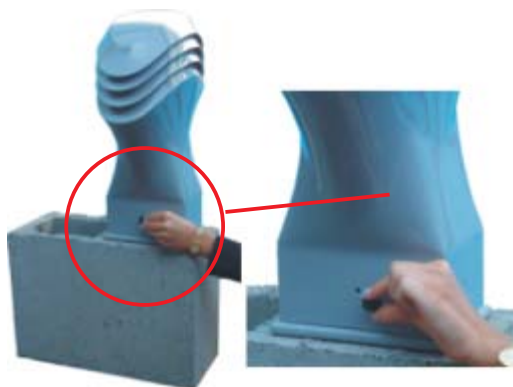
монтаж дефлектора с переходным монтажным элементом при помощи пластиковых затычек
