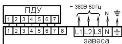
Рис. 3. Схемы подключения завес к электросети и пульта управления
