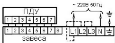
Рис. 3. Схемы подключения завес к электросети и пульта управления
